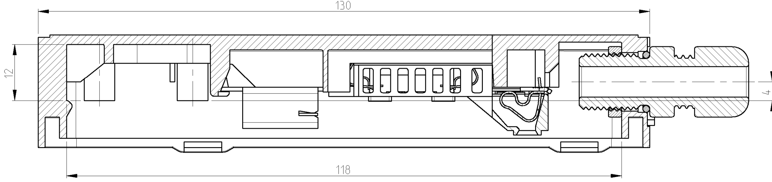
SECTION A-A SCHNITT A-A
